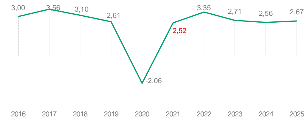
Gráfico 2. Variación interanual de la media mensual de personas afiliadas. 2016-2025
